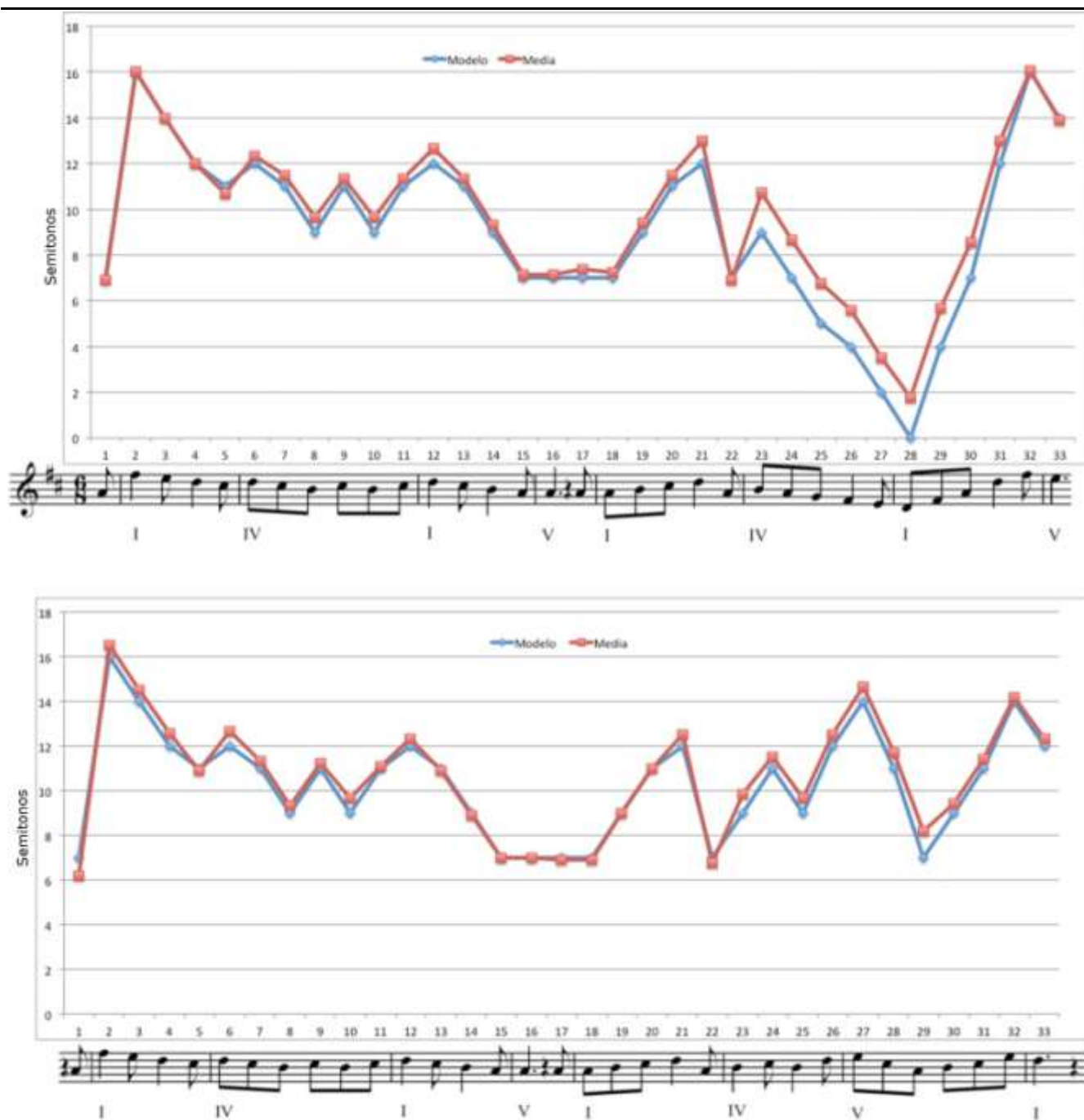
Figura 2: Gráfico comparativo entre la melodía presentada como modelo (color azul) y una media resultante de todas las ejecuciones (color rojo). El eje horizontal refiere a cada una de las notas sucesivas de la melodía, mientras que el eje vertical representa los semitonos medidos en relación a la distancia de cada nota respecto de la tónica. En el panel superior se muestra la primera frase de la melodía y en el inferior la segunda.
